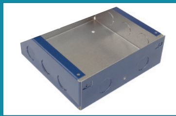
La herramienta SnapLock elimina la necesidad de aplicar soldadura por puntos en la producción de las cajas
