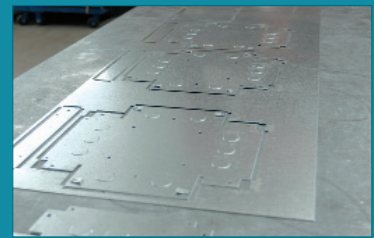
La perforación y conformación de los modelos de cajas eléctricas se realiza con rapidez en operaciones consecutivas de punzonado y plegado
