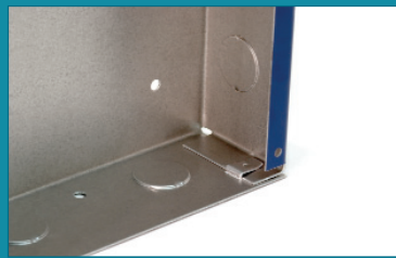
La caja eléctrica conformada obtenida con la herramienta SnapLock dispone de pestañas pulidas de enganche automático realizadas con la chapa prelacada
