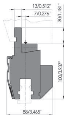
Ejemplo: Portaherramientas con adaptación ES I que incluye alineación Ty
