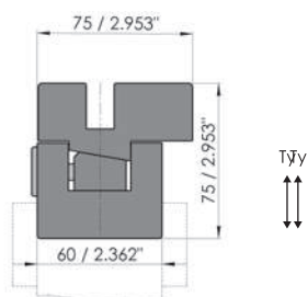
Ejemplo: Portaherramientas con adaptación ES IV que incluye alineación Ty
