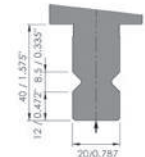
NS III Adaptación New Standard III
